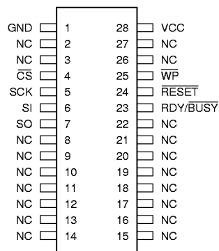
SOIC
